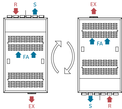
Ausrichtung der Einheit Unit orientation
