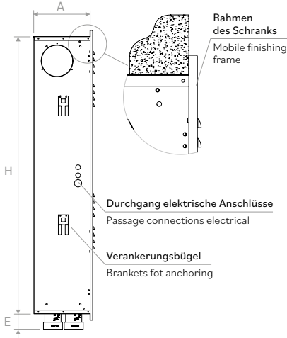
Seitenansicht | Lateral view
