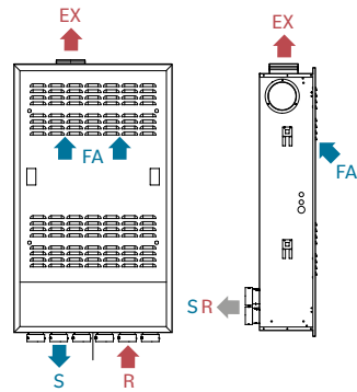
Position der Vor- und Rücklaufanschlüsse Spigots position supply/return
