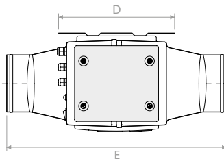
Vue latérale | Side view
