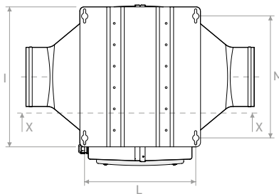
Vue de dessus | Top view
