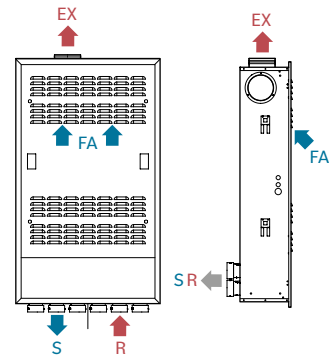
Poziționare racorduri introducere/evacuare Spigots position supply/return
