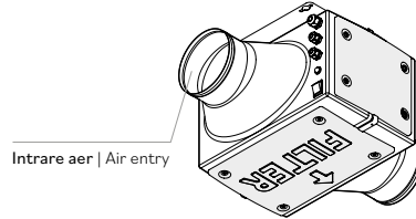
Vedere izometrică de jos Isometric bottom view
