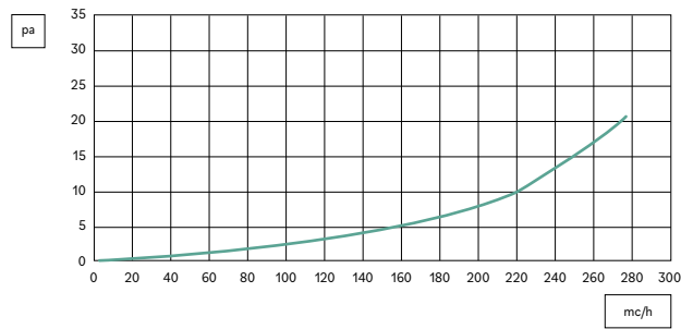
PLUGPVMCMR PIERDERE DE PRESIUNE PE UN FLUX | AIR PRESSURE DROP FOR SINGLE
